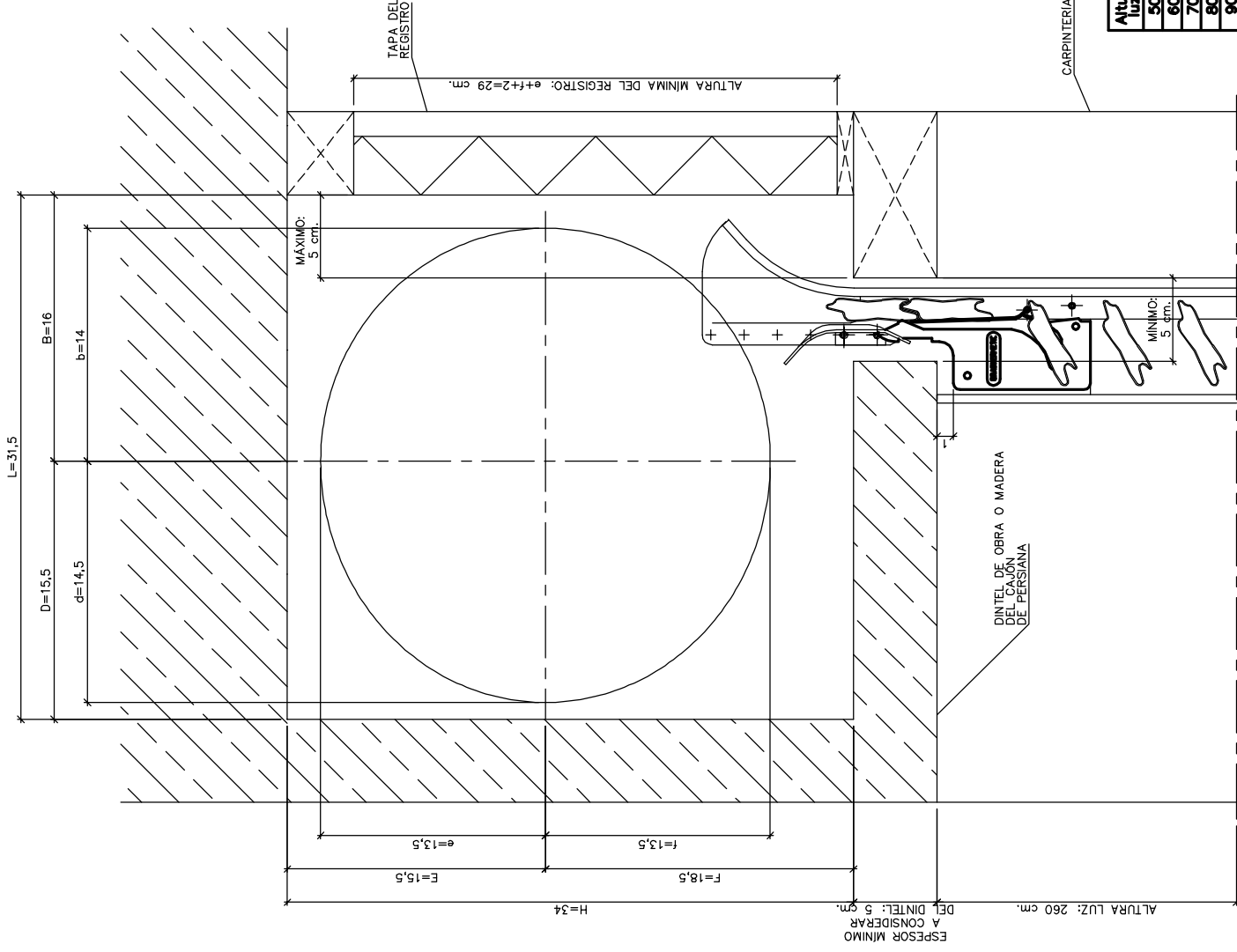
SECCIÓN PARA ALTIMA LUZ=260 cm. E:1:2
