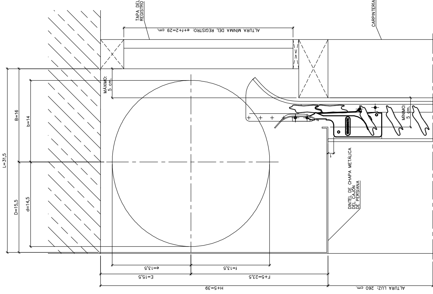
SECCIÓN PARA ALTIMA LUZ=260 cm. E:1:2
